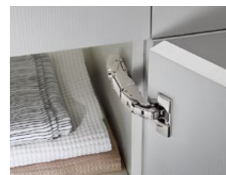
CLIP top BLUMOTION 125° для конструкцій із профільними дверцятами
