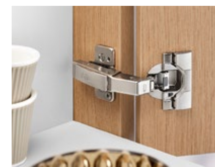
CLIP top BLUMOTION для конструкцій із фальш-панеллю
