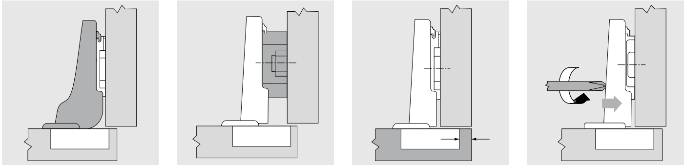
Завіси з різними вигинами плеча Висота монтажної планки Зміна відстані до чашки Регулювання за шириною
